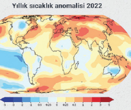
Yıllık sıcaklık anomali 2022
