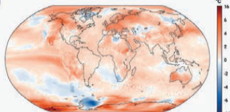
Eylül 2023 küresel sıcaklık sapması (Referans aralığı: 1991-2020)
